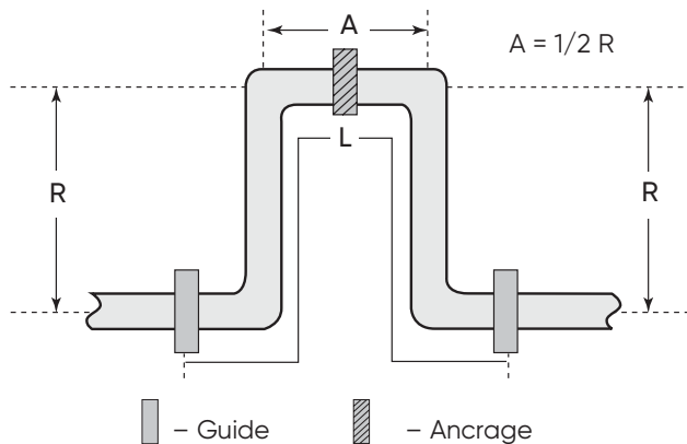
Figure 4 – Boucle de dilatation de type courant
