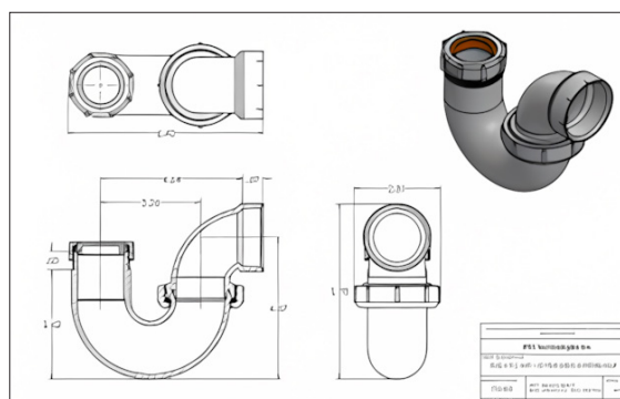
Plans dimensionnels
