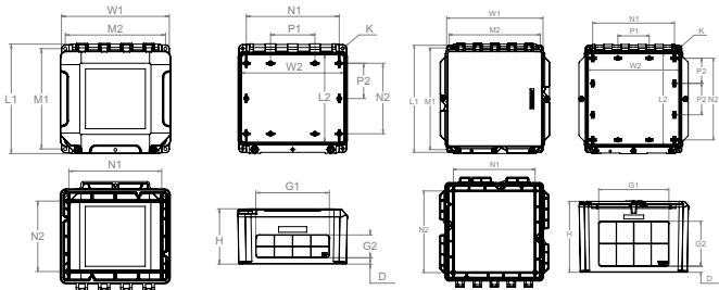
JBXH884 - JBXH887
